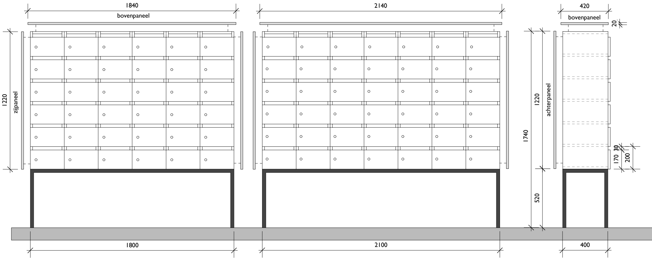
VOORAANZICHT HP1306 OS 520mm
