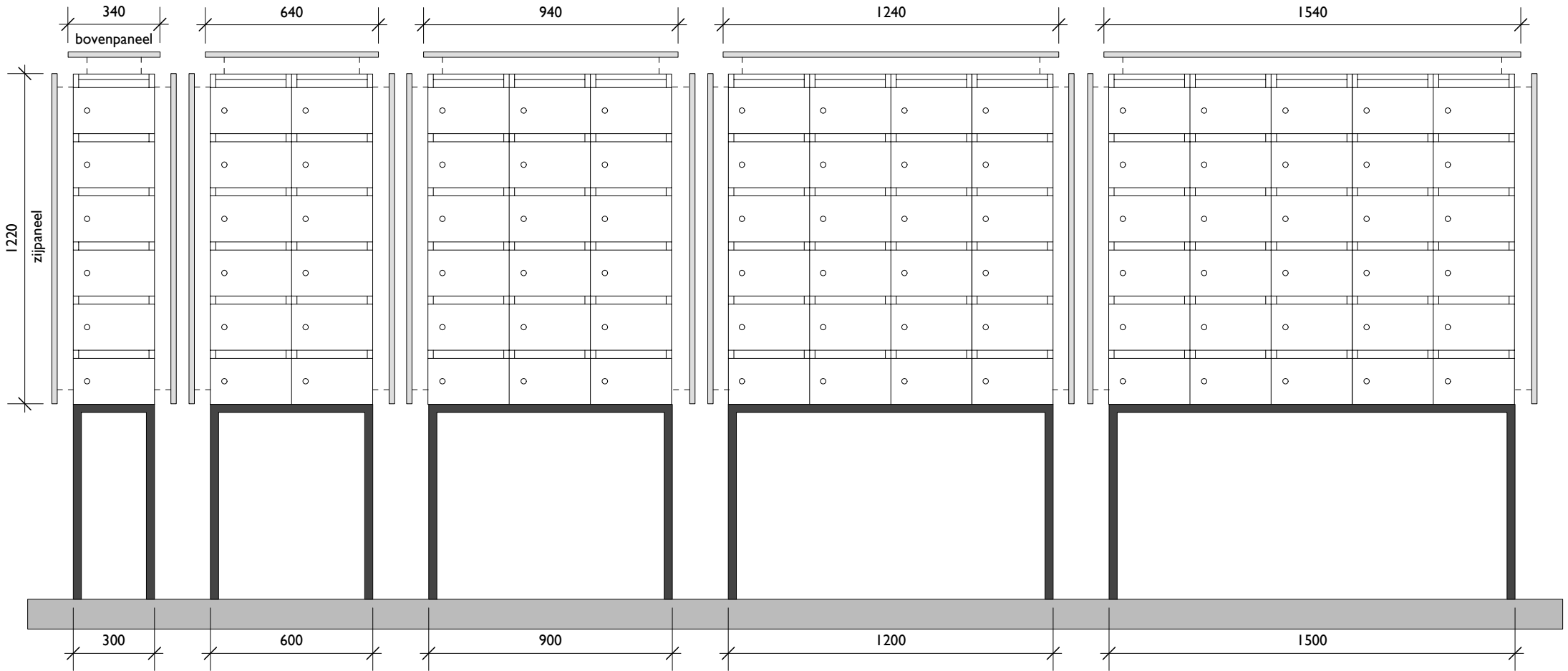
VOORAANZICHT HPI 306 OS 720mm
