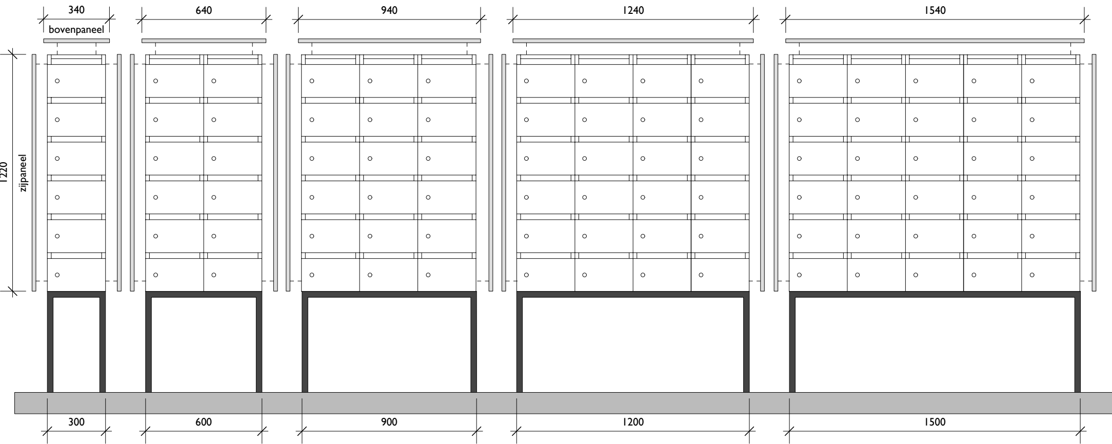
VOORAANZICHT HPI 306 OS 520mm
