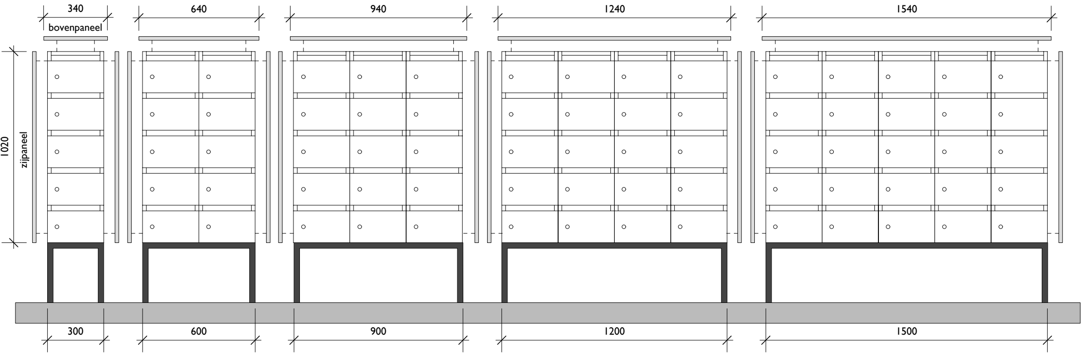
VOORAANZICHT HPI 305 OS 320mm
