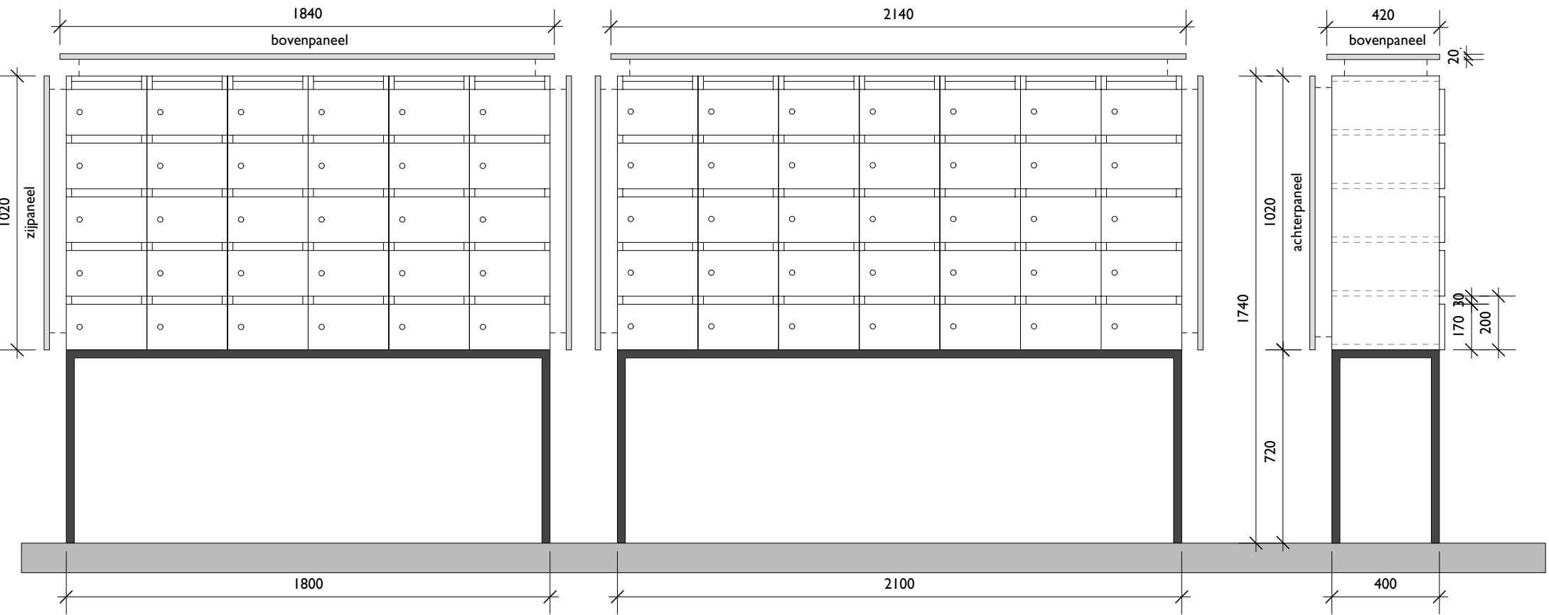
VOORAANZICHT HPI 305 OS 720mm
