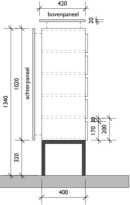
ZIJAAANZICHT HPI 305 OS 320mm
