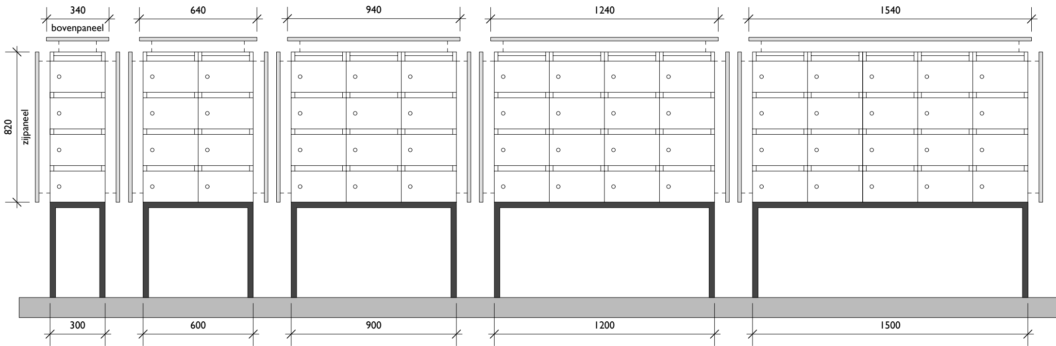
VOORAANZICHT HPI 304 OS 520mm
