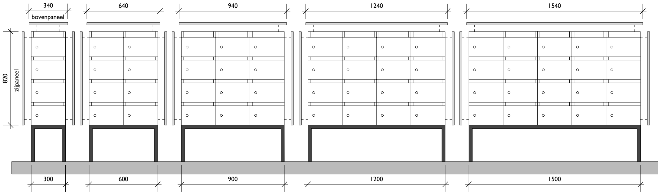
VOORAANZICHT HP1304 OS 320mm
