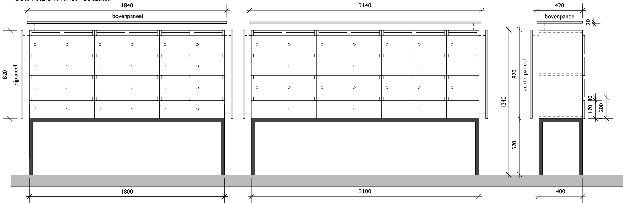
ZIJAAANZICHT HPI 304 OS 520mm
